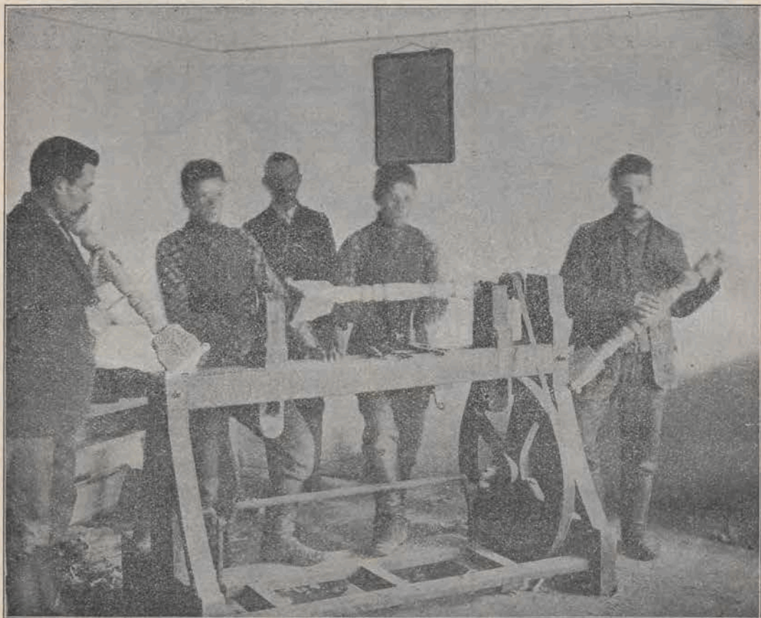
Ceglów. Warstat tokarski (str. 92).
